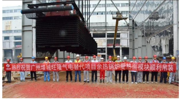
图：广州增城旺隆气电替代工程项目 1 号余热锅炉受热面模块顺利吊装
